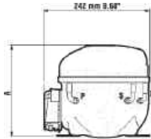
Embraco Aspera 3/4 Hp
