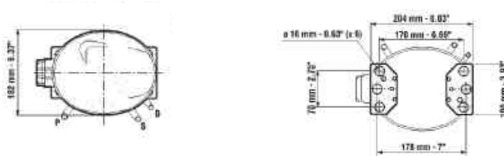
Modelo de Compresor: NE9213E
